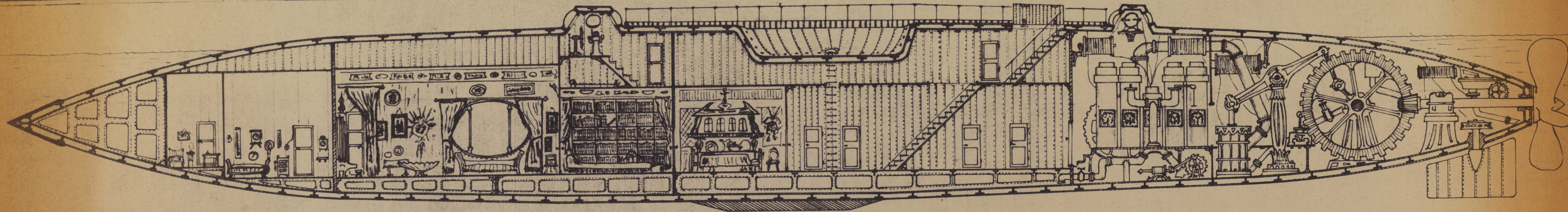
plan et coupe du sous-marin Nautilus construit sur les plans du capitaine Nemo 1865
