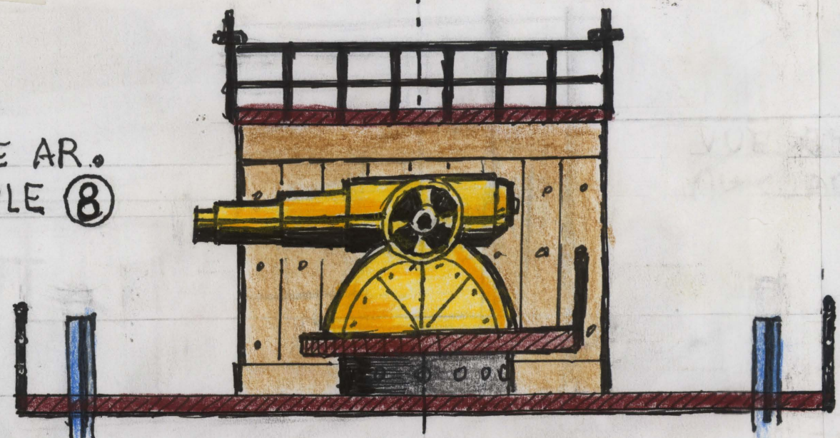
VUE AR. AU COUPLE 12
