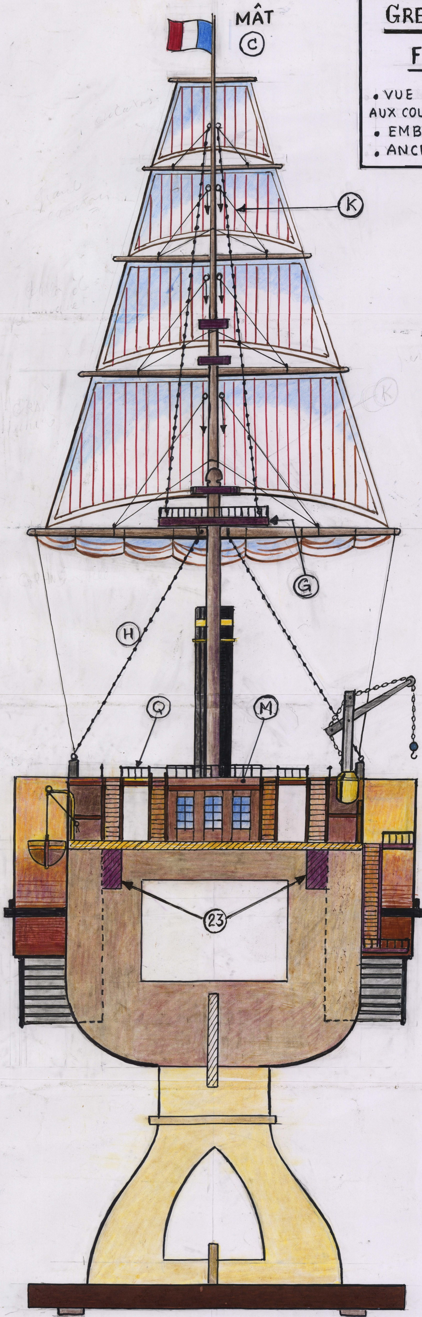
VUE AU COUPLE ⑨ AVEC PIEDS ET SOCLE
