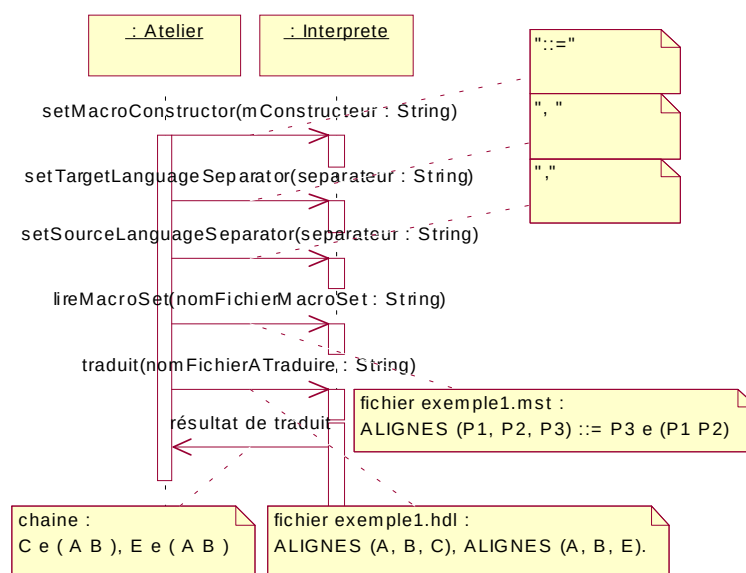
Figure 4.12 – Exemple de traduction
