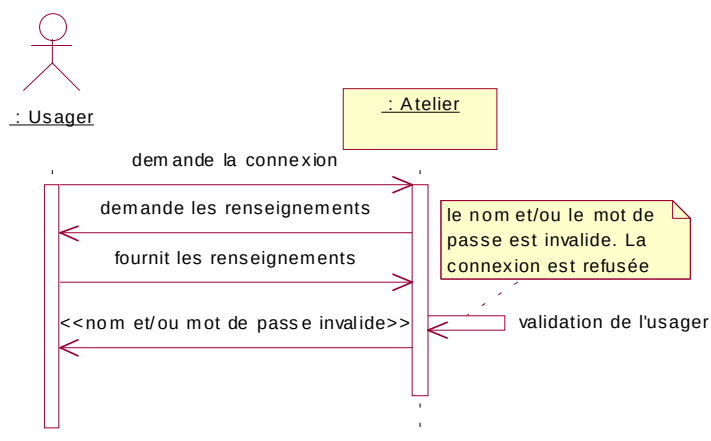
Figure 1.13 – Diagramme de séquences : connexion refusée pour renseignements incorrects
