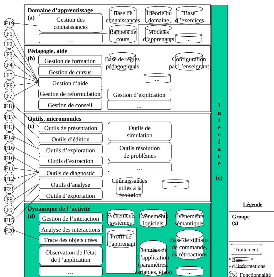
Figure 2.13 – Répartition des fonctionnalités en cinq groupes
