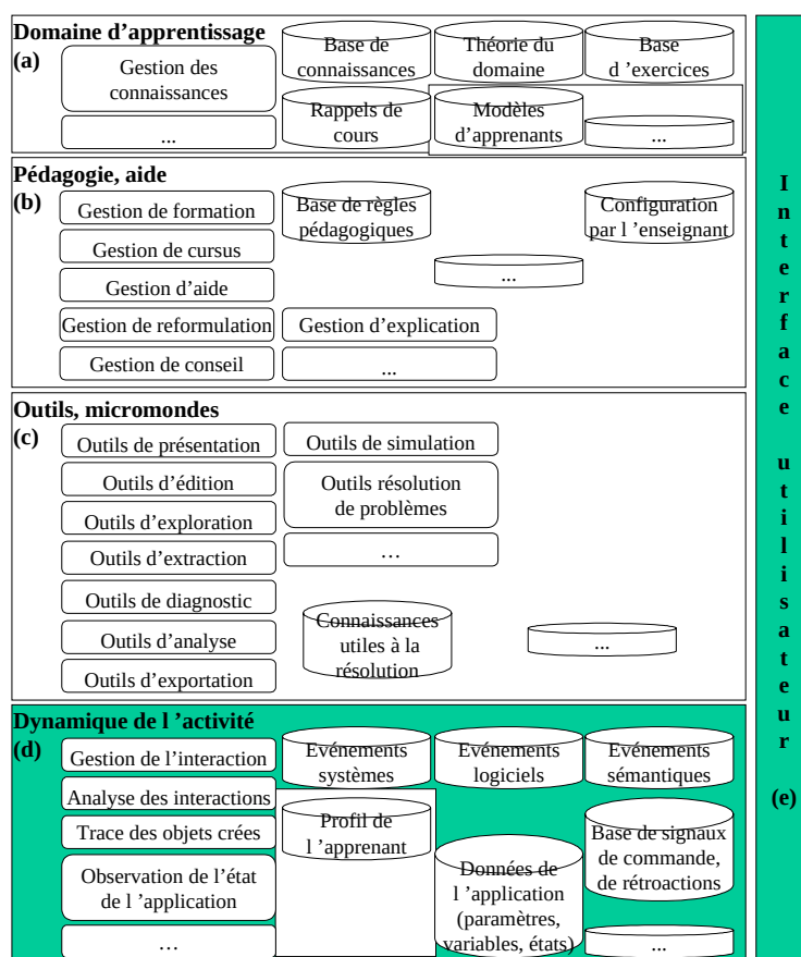
Figure 2.11 – Présentation des EIAO en cinq groupes
