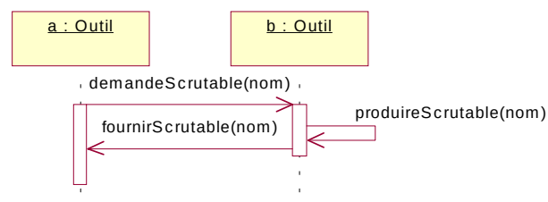
Figure 3.21 – Un outil consulte un scrutable d'un autre outil
