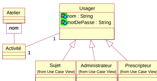
Figure 1.21 – Diagramme de classe des objets du domaine
