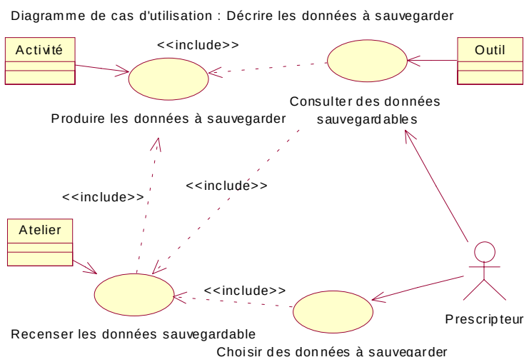
Figure 3.22 – Diagramme de cas d'utilisation : Décrire les données à sauvegarder
