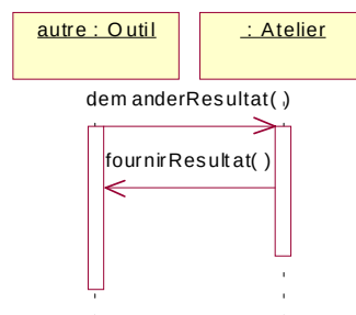
Figure 3.15 – Diagramme de séquence : un objet consulte un résultat
