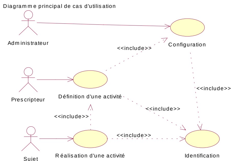
Figure 1.11 – Diagramme principal des cas d'utilisation
