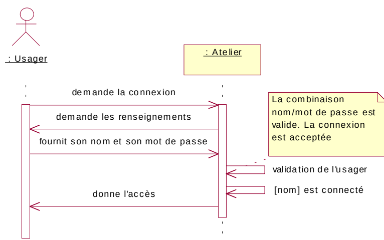
Figure 1.12 – Diagramme de séquences : connexion acceptée
