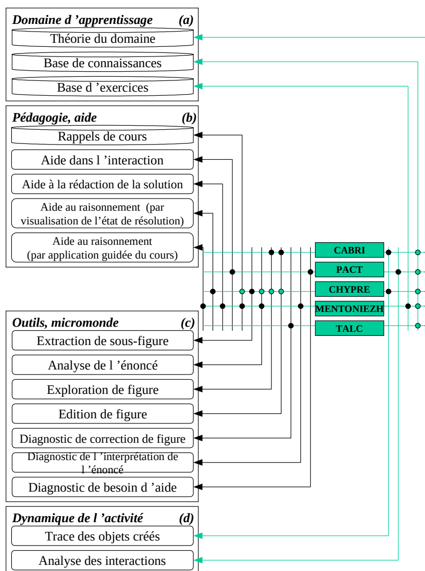
Figure 1.8 – Fonctionnalités des EIAO de l'exemple introductif
