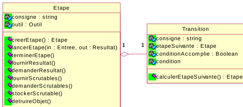
Figure 4.8 – Les classes Etape et Transition
