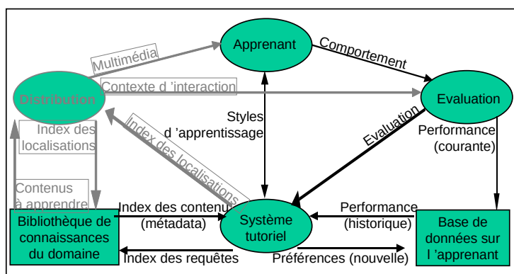
Figure 2.8 – Le processus «Distribution» de l'architecture LTSA
