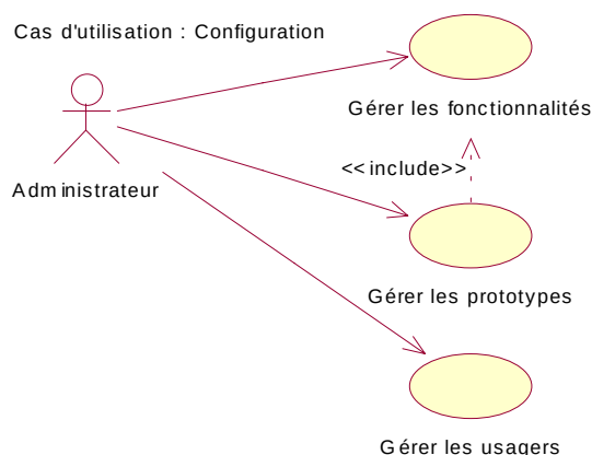
Figure 1.16 – Diagramme de cas d'utilisation : configuration
