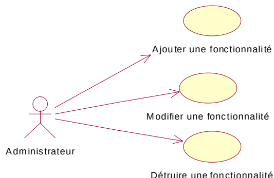
Figure 1.20 – Diagramme de cas d'utilisation : gérer la liste des fonctionnalités
