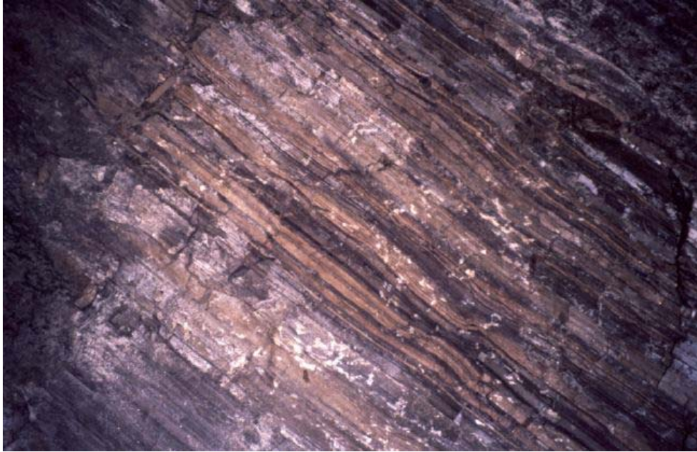
Figure 11 : alternance de lamines parallèles sombres et claires dans la mine (photo T. Mongenot)
