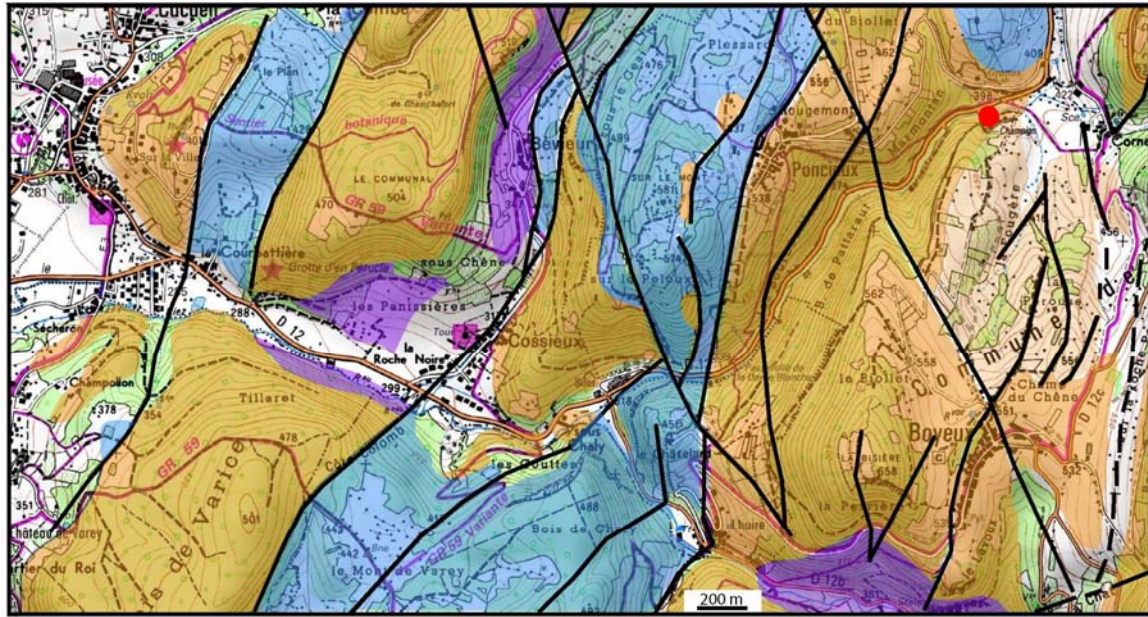
Figure 20 : localisation de l'ancienne carrière souterraine de Cornelle (rond rouge). L'entrée de la grotte de Jujurieux est repérée par une étoile rouge à gauche.
