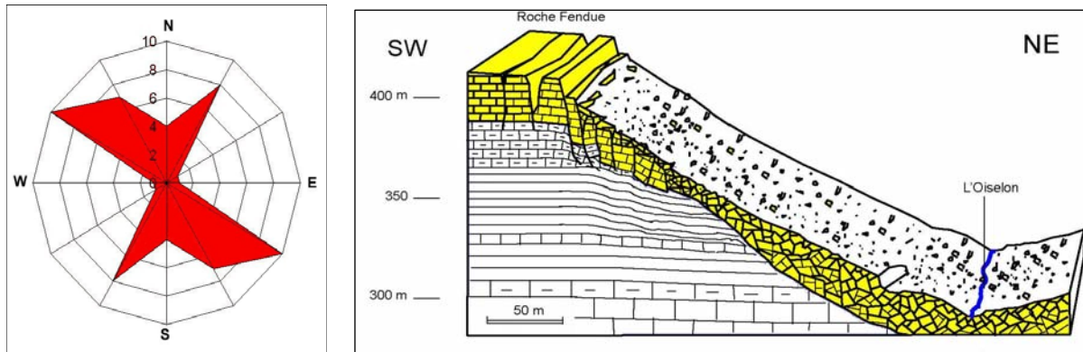
Figure 17 : fracturation au Nord des Barmes : deux faisceaux principaux perpendiculaires Figure 18 : coupe NNE-SSW de la bordure nord du plateau des Barmes.
