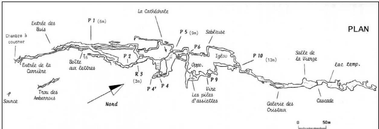
Figure 32 : le réseau souterrain de la grotte de Jujurieux (d'après Chirol, 2000).
