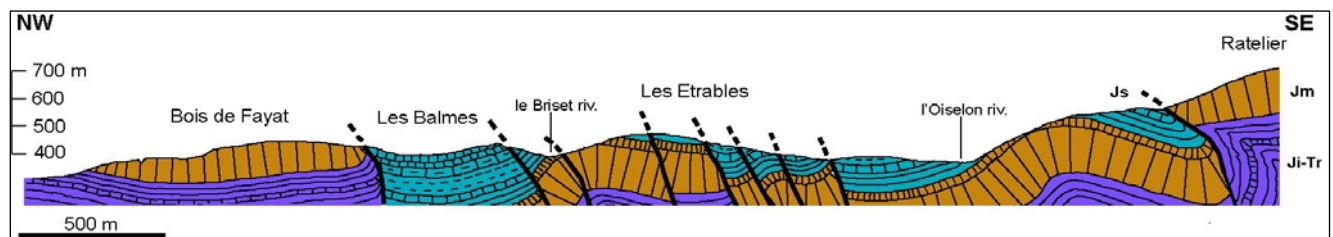
Figure 19 : coupe NW-SE dans l'extrait de carte ci-dessus.
